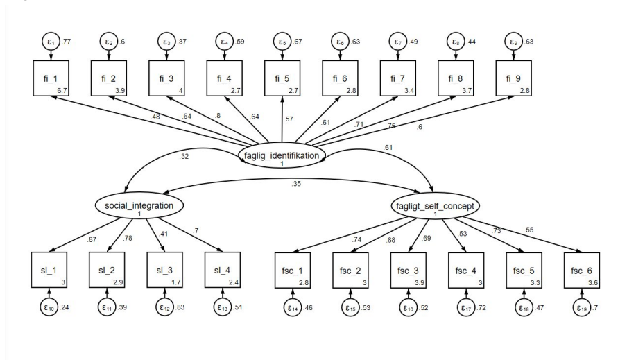
Figur 1: CFA-model.
