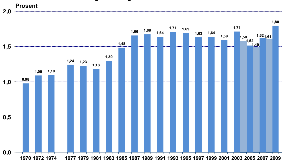
FoU-utgifter i Norge som andel av BNP 1970-2009.
